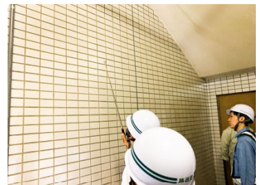
点検ハンマーによる打音調査
