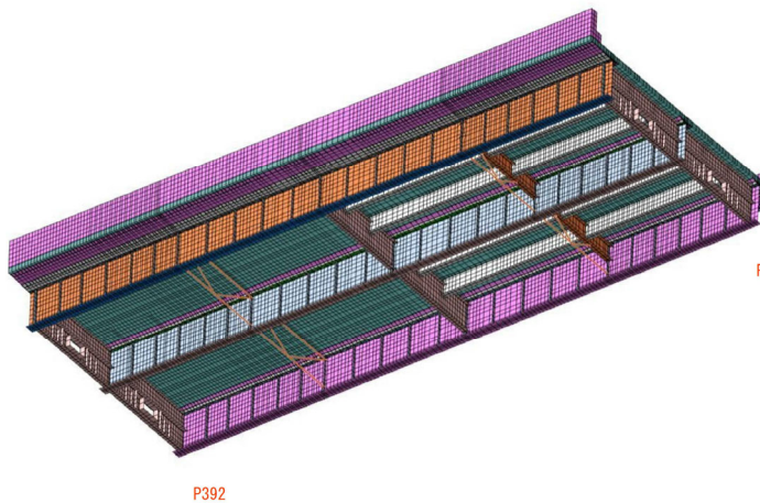
解析に用いた全橋 FEM モデル
