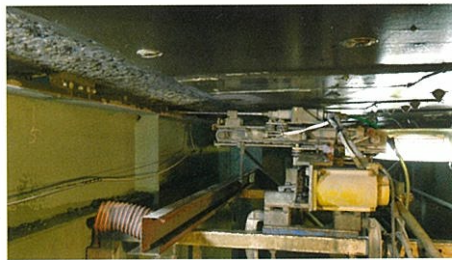
ウォータージェットによるハンチ除去
