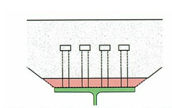
ハンチ除去の範囲
