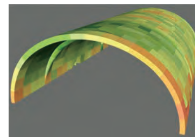
「Dynamo」用いたCIMモデル作成(トンネル覆工厚出形確認)
